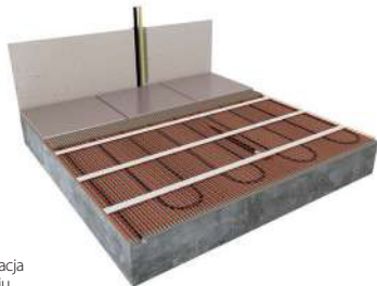
Instalacja w wylewce
