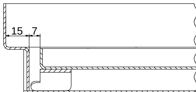
PRZEKRÓJ WZDŁUŻNY (PURE)
