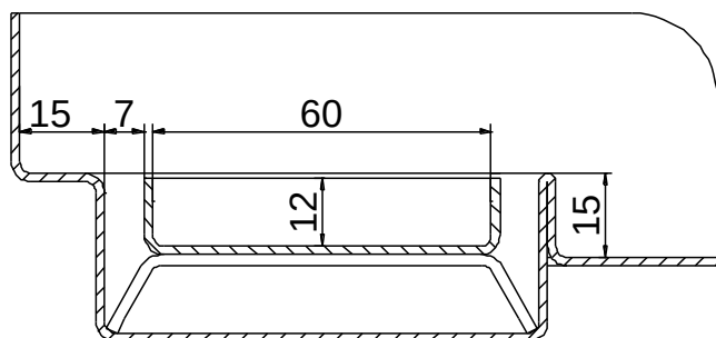
PRZEKRÓJ POPRZECZNY (PURE)
